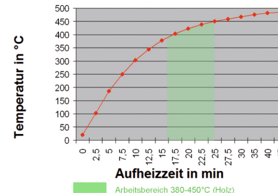
Aufheizdiagramm T1-400-12540
